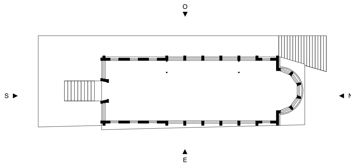
PLAN RDC
