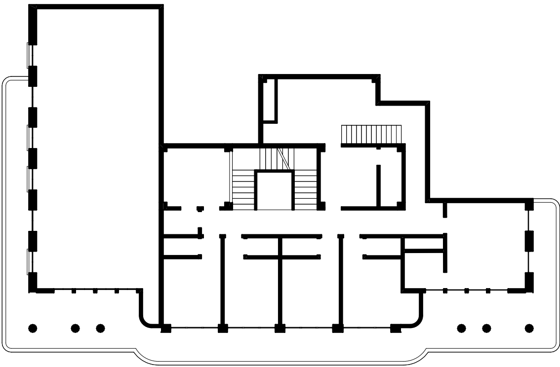
PLAN R+2
