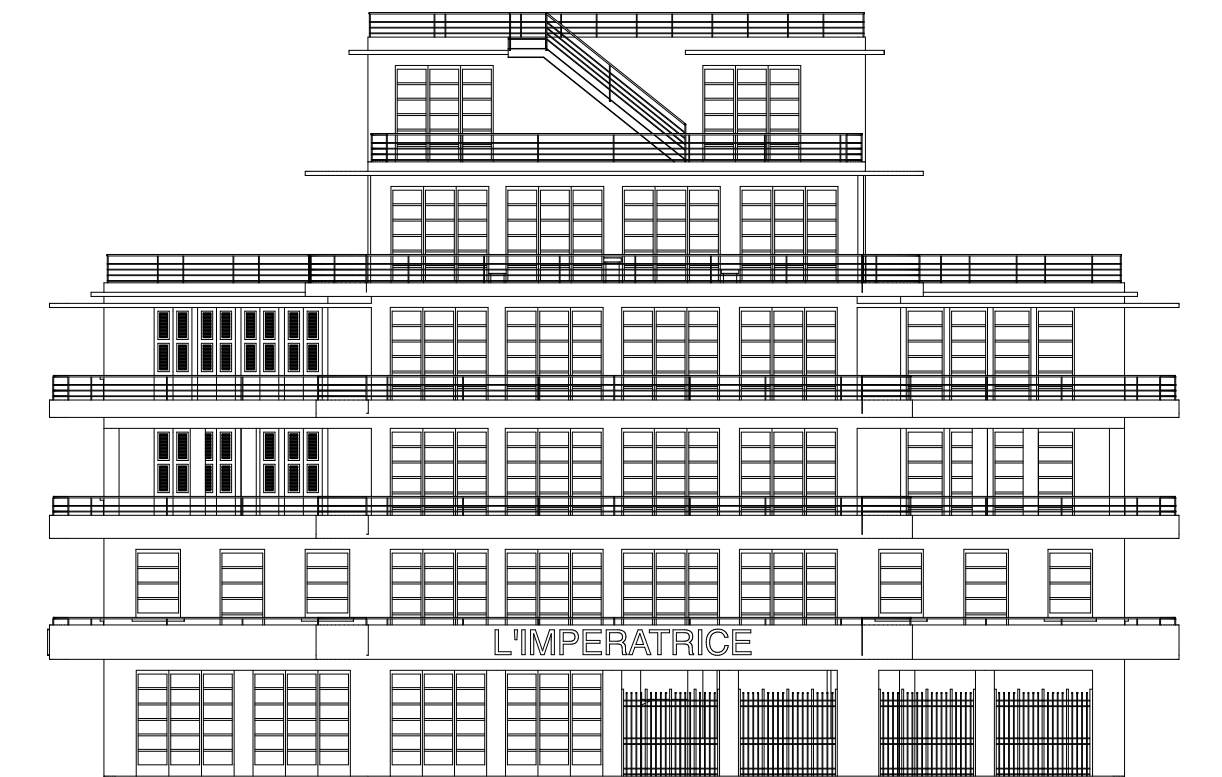
FAÇADE EST
