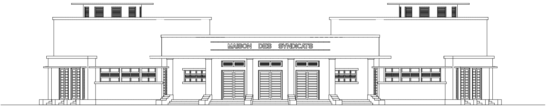
FAÇADE SUD
