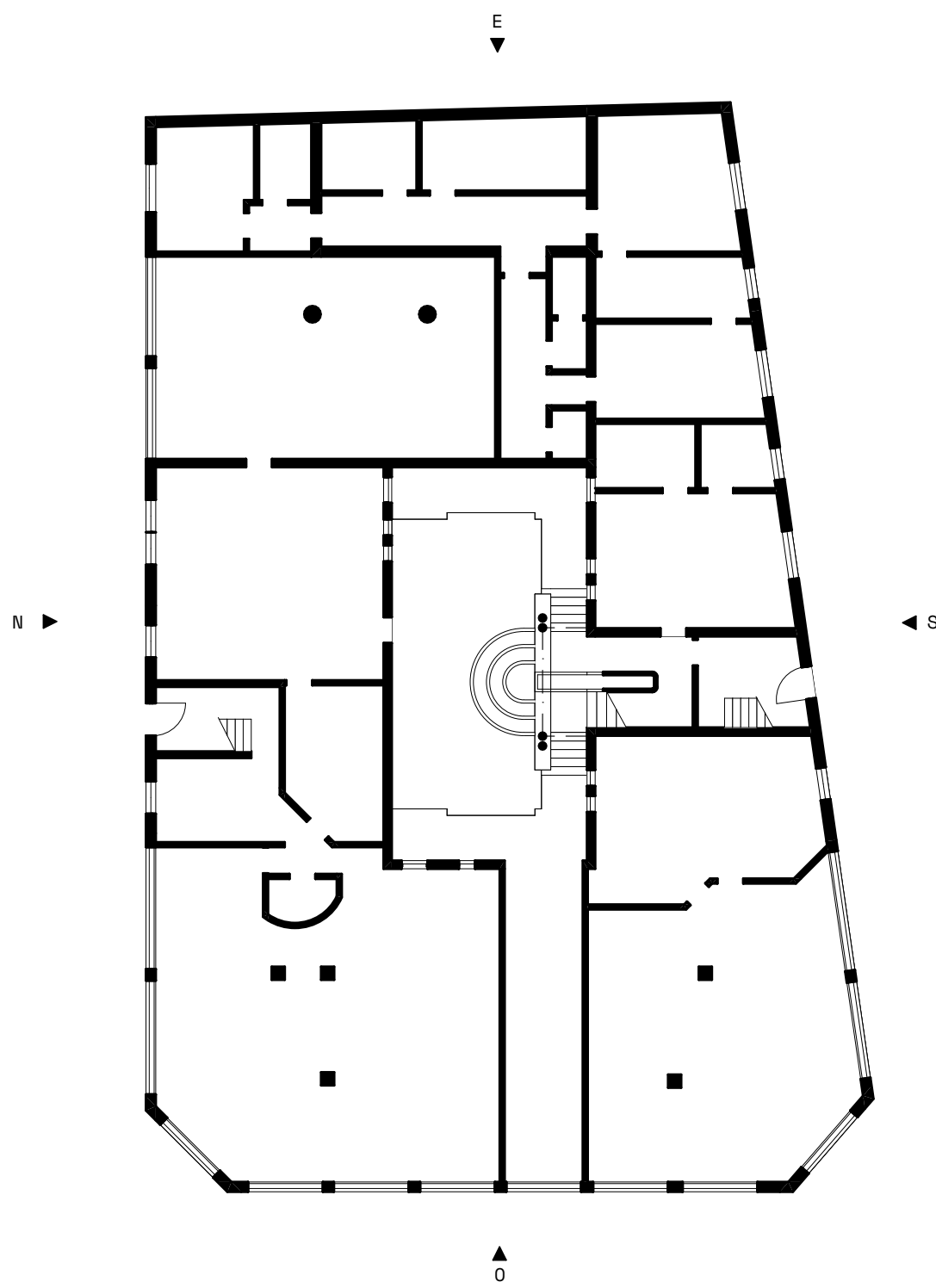
PLAN RDC
