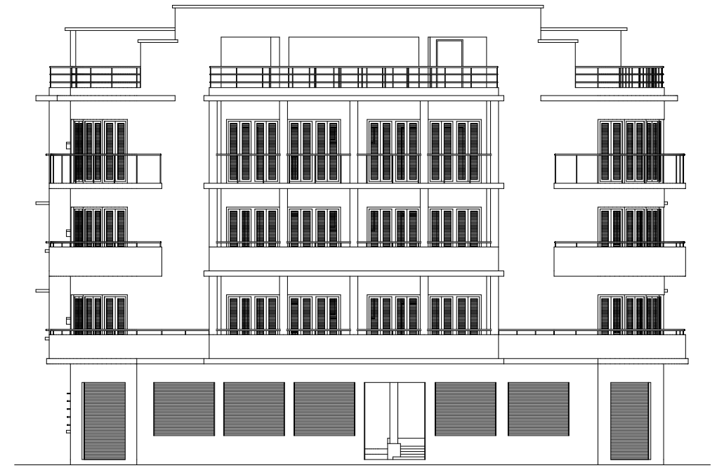
FAÇADE OUEST
