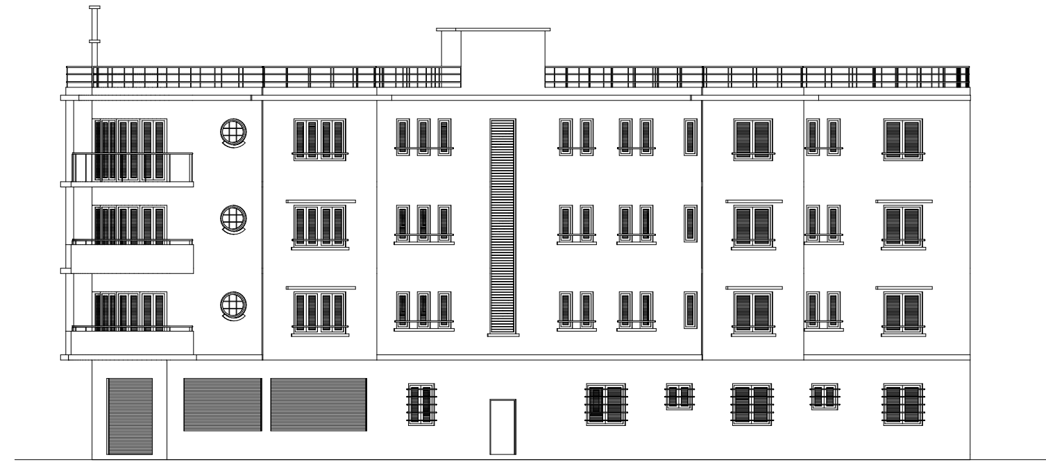
FAÇADE SUD
