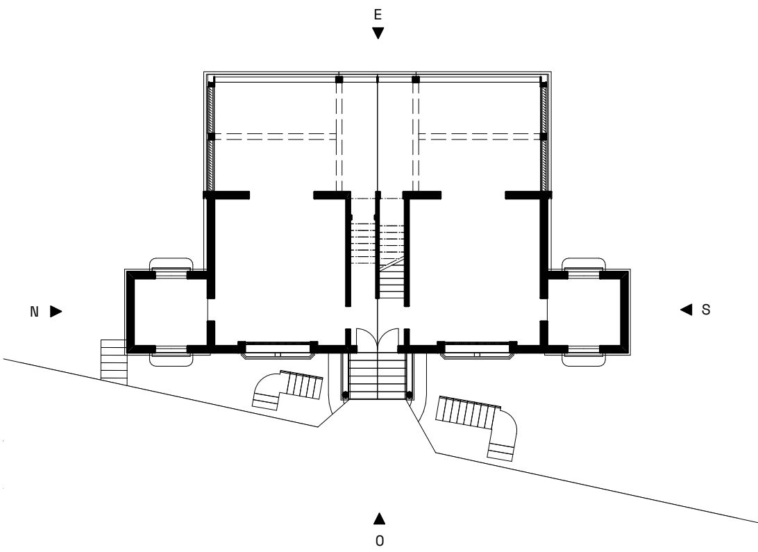
PLAN RDC
