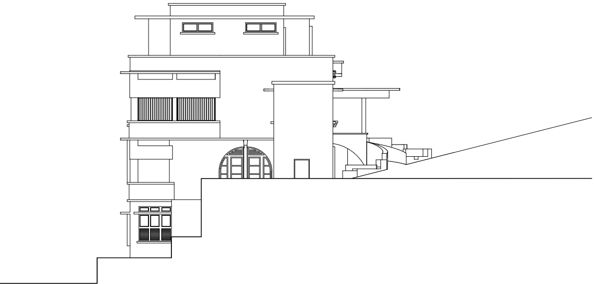
FAÇADE NORD
